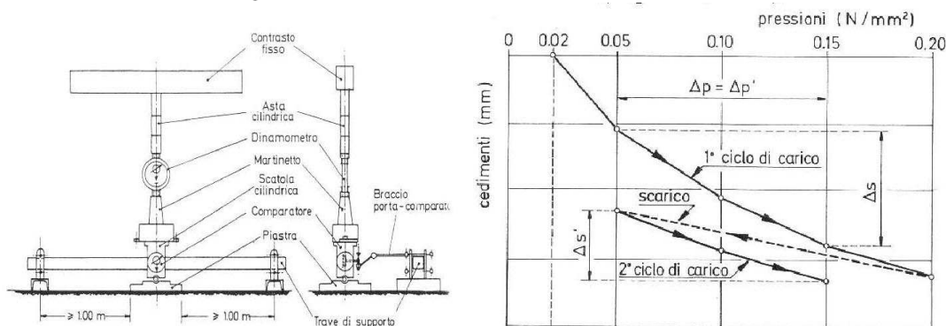
Figura 6 -Piastra di carico e strati di sottofondo
