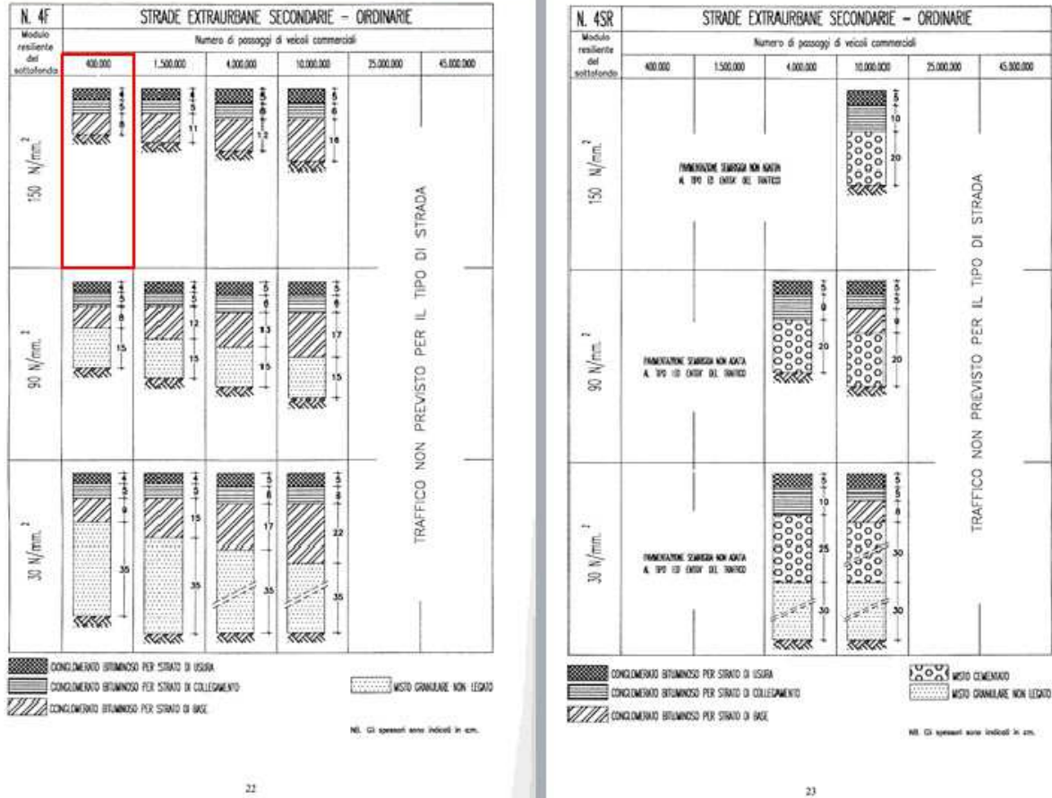
Figura 8 - Scheda n. 4F del Catalogo delle Pavimentazioni
